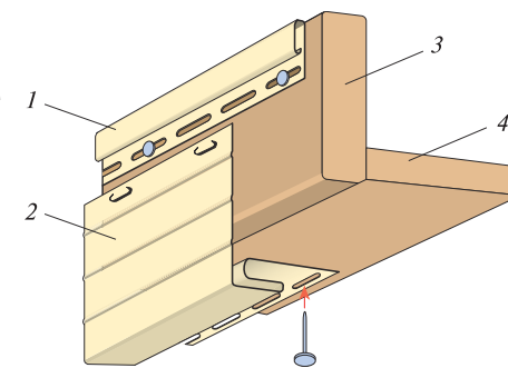
Рис. 55. Крепление целой J-фаски к причелине: 1 — финишный профиль; 2 — J-фаска; 3 — причелина; 4 — деревянная обшивка карниза
