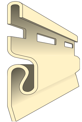
Рис. 2. Антиураганный замок сайдинга Дёске
