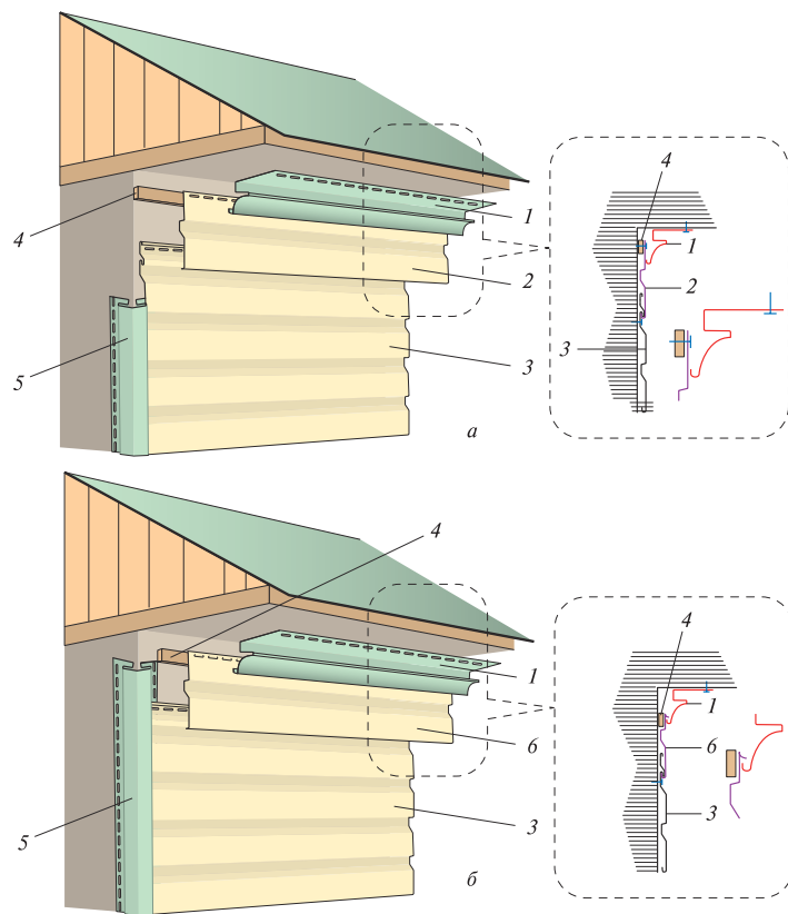
Рис. 39. Схема монтажа сайдинга прикрываемых молдингом Döcke: а – на крепежах; б – на зацепах; 1 – молдинг Döcke; 2 – подкарнизный сайдинг с дополнительными гвоздевыми отверстиями; 3 – рядовой сайдинг; 4 – выравнивающая рейка; 5 – угловой сайдинг; 6 – подкарнизный сайдинг с «зацепами»
