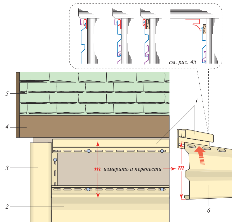
Рис. 38. Установка сайдинга на «зацепах» под карнизом или соффитом: 1 – завершающие профили (финишный профиль на выравнивающей рейке или внутри J-профиля (или наличника), либо молдинг Döcke); 2 – рядовая сайдинговая панель; 3 – угловой профиль; 4 – карниз; 5 – крыша; 6 – подкарнизная (резаная) сайдинговая панель с зацепами
