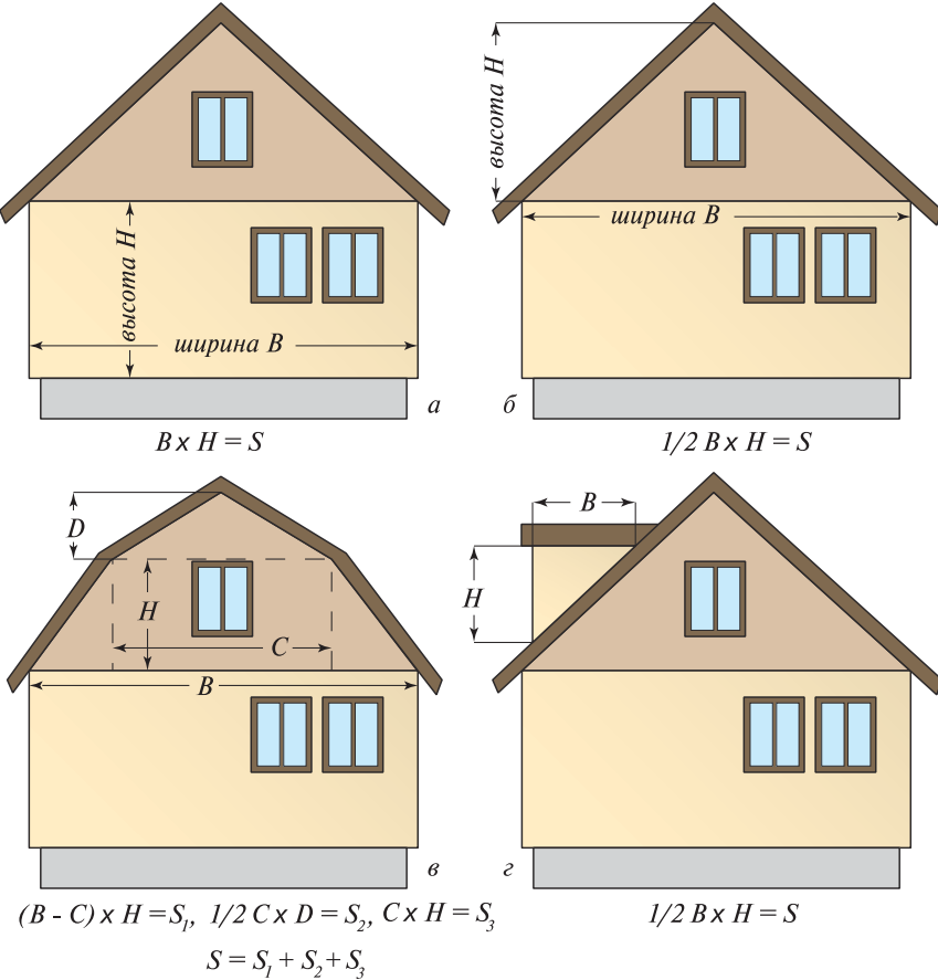
Рис. 6. Расчет площадей рядового сайдинга: а — по стенам; б — по треугольным фронтонам; в — по ломанным фронтонам; г — по слуховым и чердачным окнам
