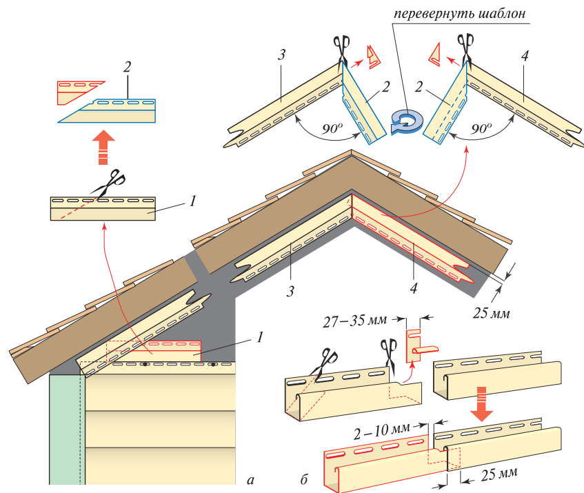
Рис. 41. Установка J-профиля на щипец: а — вырезание шаблона и установка J-профиля; б — стыкование J-профиля по длине; 1 — обрезок J-профиля; 2 — шаблон; 3 — левый элемент обшивки; 4 — то же, правый
