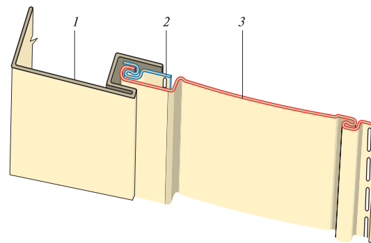
Рис. 48. Вариант узла примыкания вертикального сайдинга к угловому профилю с установкой стартового профиля: 1 — принимающий профиль; 2 — стартовый профиль; 3 — вертикальный сайдинг
