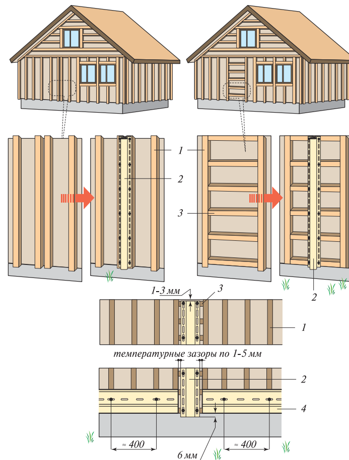
Рис. 28. Установка Н-профилей: 1 — вертикальная обрешетка; 2 — Н-профиль; 3 — горизонтальная обрешетка; 4 — стартовый профиль
