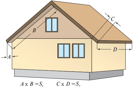
Рис. 7. Расчет площадей софмитов
