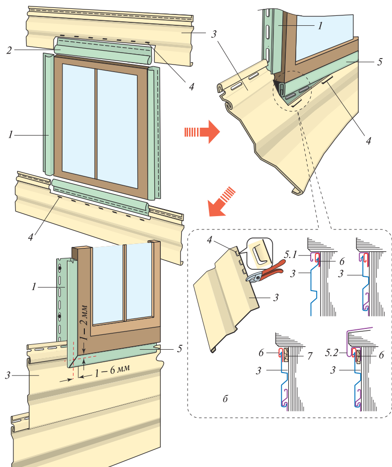
Рис. 35. Установка сайдинга вокруг проемов на «зацепах»: а – общая схема монтажа; б – варианты узлов нижней (и верхней) обвязки; 1 – боковой профиль обвязки проема (J-профиль, наличник или околонный профиль); 2 – верхний профиль обвязки; 3 – рядовая сайдинговая панель; 4 – зацеты; 5 – нижний профиль обвязки (5.1 – J-профиль или наличник, 5.2 – околонный профиль); 6 – финишный профиль; 7 – выравнивающая высота деревянная рейка
