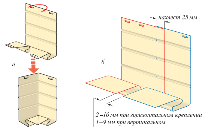
Рис. 56. Загибание (а) и нахлест (б) J-фасок Döcke
