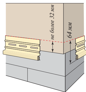
Рис. 17. Нанесение обшивки на цоколь
