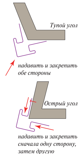
Рис. 21. Монтаж угловых профилей на не прямоугольные углы
