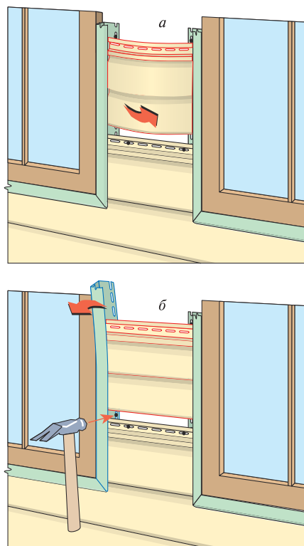
Рис. 37. Установка сайдинга в узких местах: а – сгибанием; 2 – с отрывом обрамляющего профиля
