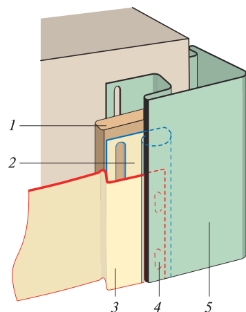
Рис. 46. Вариант узла примыкания вертикального сайдинга к угловому профилю: 1 — деревянная выравнивающая высота рейка; 2 — J-профиль; 3 — вертикальный сайдинг; 4 — зацепы; 5 — угловой профиль
