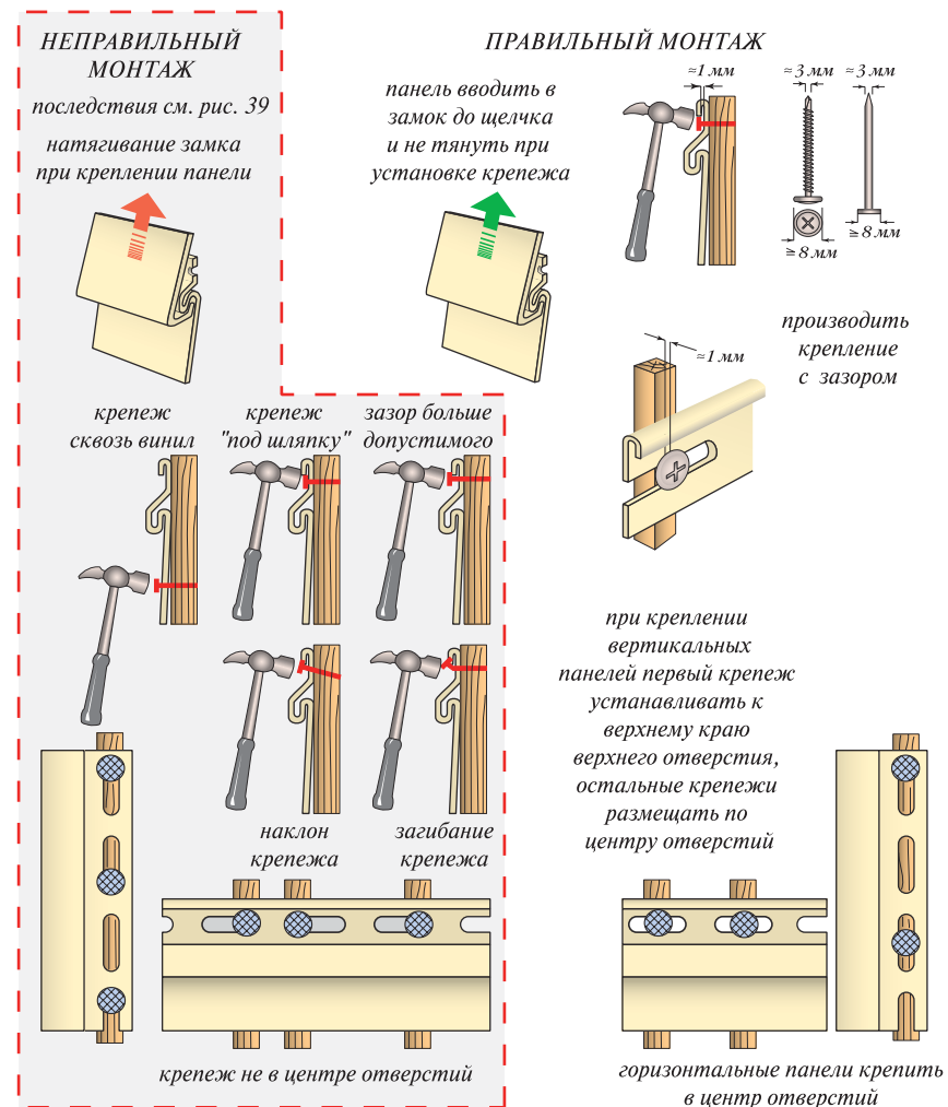
Рис. 12. Правила крепления виниловых панелей
