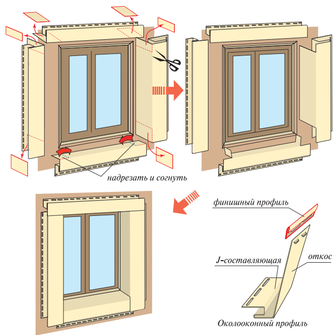
Рис. 24. Обрамление оконных и дверных проемов околооконными профилями
