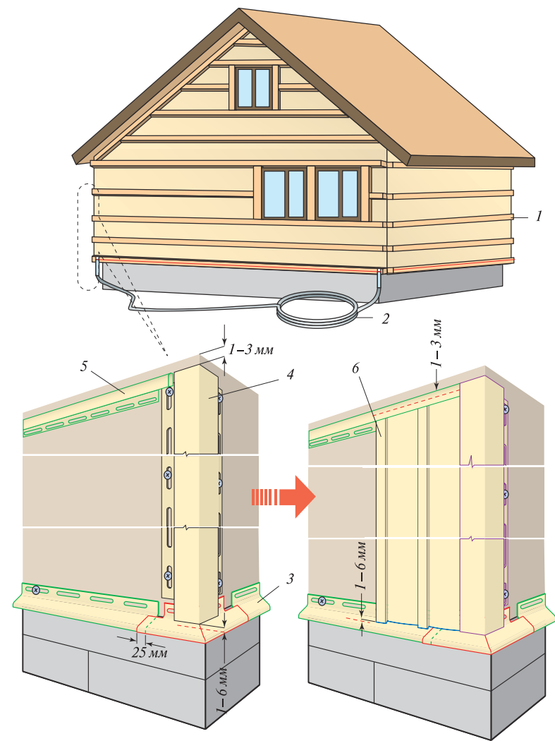
Рис. 45. Схема монтажа вертикального сайдинга: 1 — горизонтальная обрешетка; 2 — водяной уровень; 3 — отлив Дёске; 4 — угловой профиль; 5 — J-профиль; 6 — вертикальный сайдинг (неперфорированный софит)
