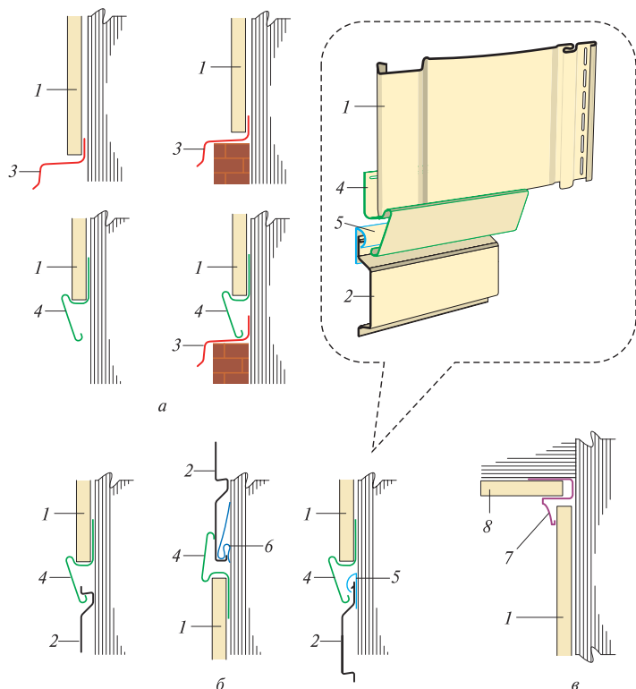
Рис. 50. Варианты расположения и стыканий сайдингов по вертикали: а — монтаж вертикального сайдинга; б — стыкование вертикальных сайдингов через профили; в — стыкование вертикальных сайдингов с софитом с использованием молдинга; 1 — вертикальный сайдинг; 2 — горизонтальный сайдинг; 3 — отлив; 4 — окантовочный профиль; 5 — финишный профиль; 6 — стартовый профиль; 7 — молдинг; 8 — софит
