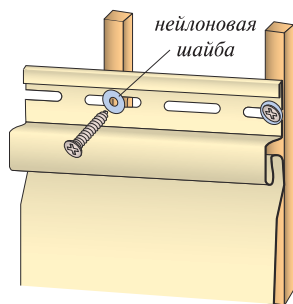
Рис. 13. Крепление сайдинга при сильных ветрах
