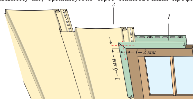
Рис. 49. Примыкания вертикального сайдинга к обрамлениям проемов: 1 — принимающий профиль; 2 — вертикальный сайдинг
