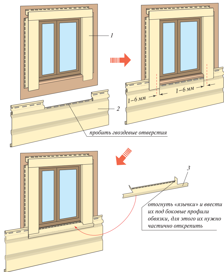
Рис. 36. Установка сайдинга вокруг проемов на обычных крепежах (гвоздях или саморезах): 1 – обвязка окна околонным профилем; 2 – рядовая сайдинговая панель; 3 – отлив Döcke
