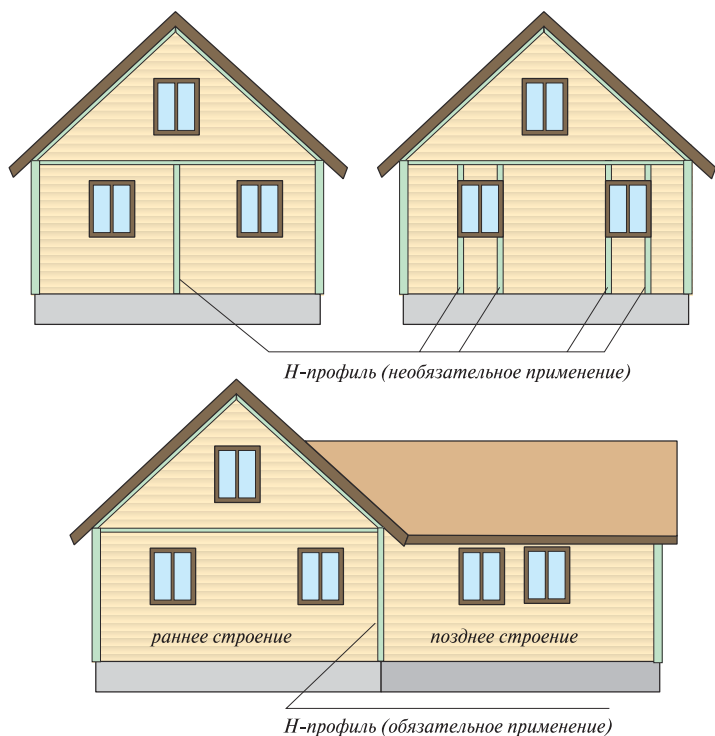
Рис. 29. Пример размещения H-профилей на фасадах
