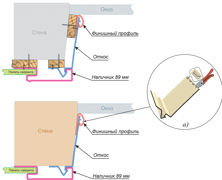
Рис. 27. Схема монтажа наличника и откоса Döcke
