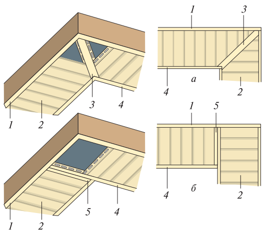
Рис. 53. Соединение софпитных подшивок на углах: а — на косой угол; б — на прямой угол; 1 — карнизный принимающий профиль; 2 — софпит; 3 — Н-профиль или два J-профиля; 4 — пристенный принимающий профиль; 5 — J-профиль
