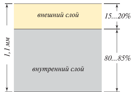
Рис. 1. Сайдинг Дёске в разрезе
