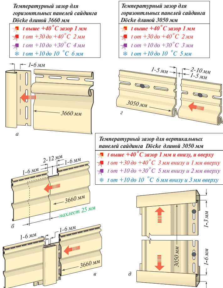
Рис. 14. Температурные зазоры на характерных узлах виниловой обшивки: а — стыкование горизонтального элемента с вертикальным (внешним или внутренним углом, J-профилем и т. п.); б — стыкование горизонтальных элементов внахлест; в — стыкование горизонтальных элементов на Н-профиле (двух J-профилях и т. п.); г — стыкование горизонтальных скрытых элементов, например, стартовой полосы; д — стыкование вертикального элемента (любого) с горизонтальным (любым).
