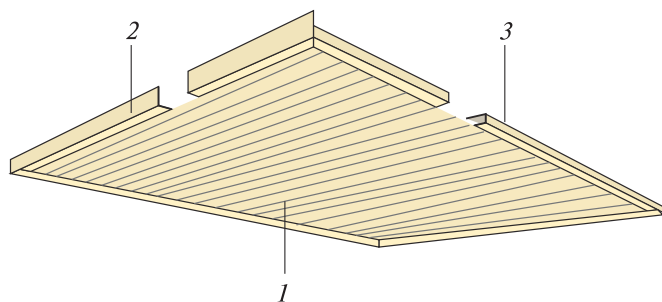
Рис. 54. Пример устройства софпита над открытой верандой: 1 — софпит; 2 — фаска; 3 — J-профиль или молдинг
